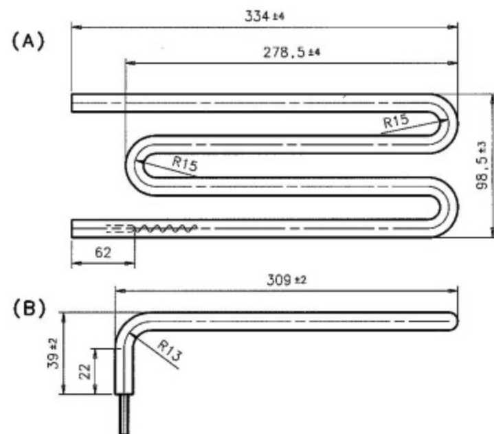
SCHEMA DI PIEGATURA ELEMENTO NON SAGOMATO
