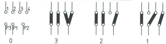
Schaltschema bei Rechtsdrehung
