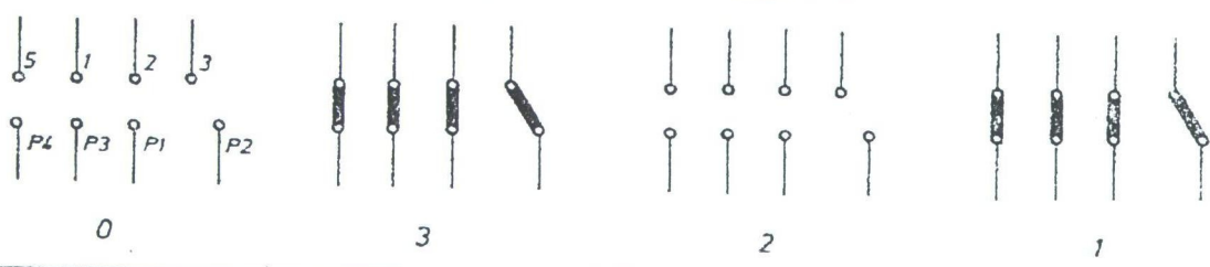
Schaltschema bei Rechtsdrehung
